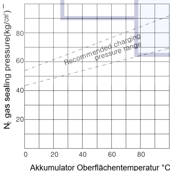
Umrechnungstabelle für die Befüllung N 2 -Gasdruck am Akkumulator
